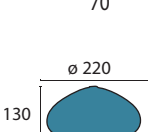
Glas 415 klar-Schliff (mit Mittelloch) Ø 220 mm, H 130 mm klar Griffrand 100 mm Öffnung oben 10 mm
