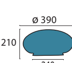
Glas 337 champ glänzend Ø 390 mm, H 210 mm champagne glänzend Griffrand 240 mm
