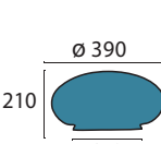
Glas 337 opal glänzend Ø 390 mm, H 210 mm opal glänzend Griffrand 240 mm
