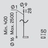
71-8263-05-05 ■ Linear end connector | Conector lineal final | Connecteur linéaire fina
