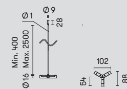
71-8257-05-05 ■ Y connector | Conector Y | Connecteur Y
