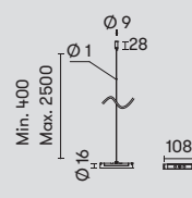
71-8262-05-05 ■ Linear connector | Conector lineal | Connecteur linéaire
