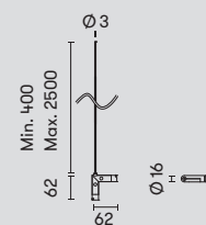
71-8255-05-05 ■ 90° vertical connector | Conector 90° vertical | Connecteur 90° vertical
