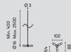
71-8251-05-05 ■ Y connector | Conector Y | Connecteur Y
