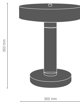
DEFEZA lampa gabinetowa 230V | Moduł LED FLM 170 mm 3000K | 23W
