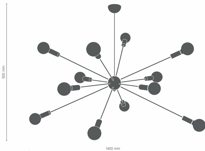
DANAIA lampa wisząca 12 pł. 12 x LED 4W E27 230V
