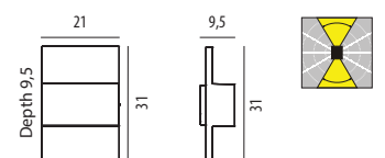
Art. 874 Art. 879 Art. 5108*
