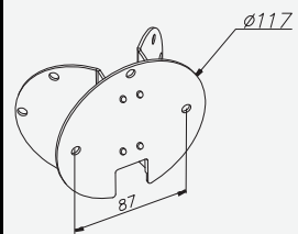
Art. 153 Corner bracket Art: 230 Art: 240 Art: 270 Art: 280, 286 Art: 290 Art: 690 Art: 1920
